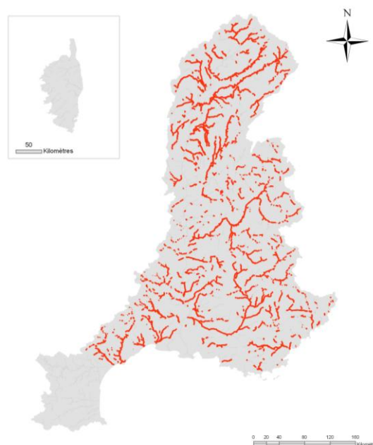
Figure 32. Réseau hydrographique où l'érosion latérale potentielle peut être prédite par SIG.
