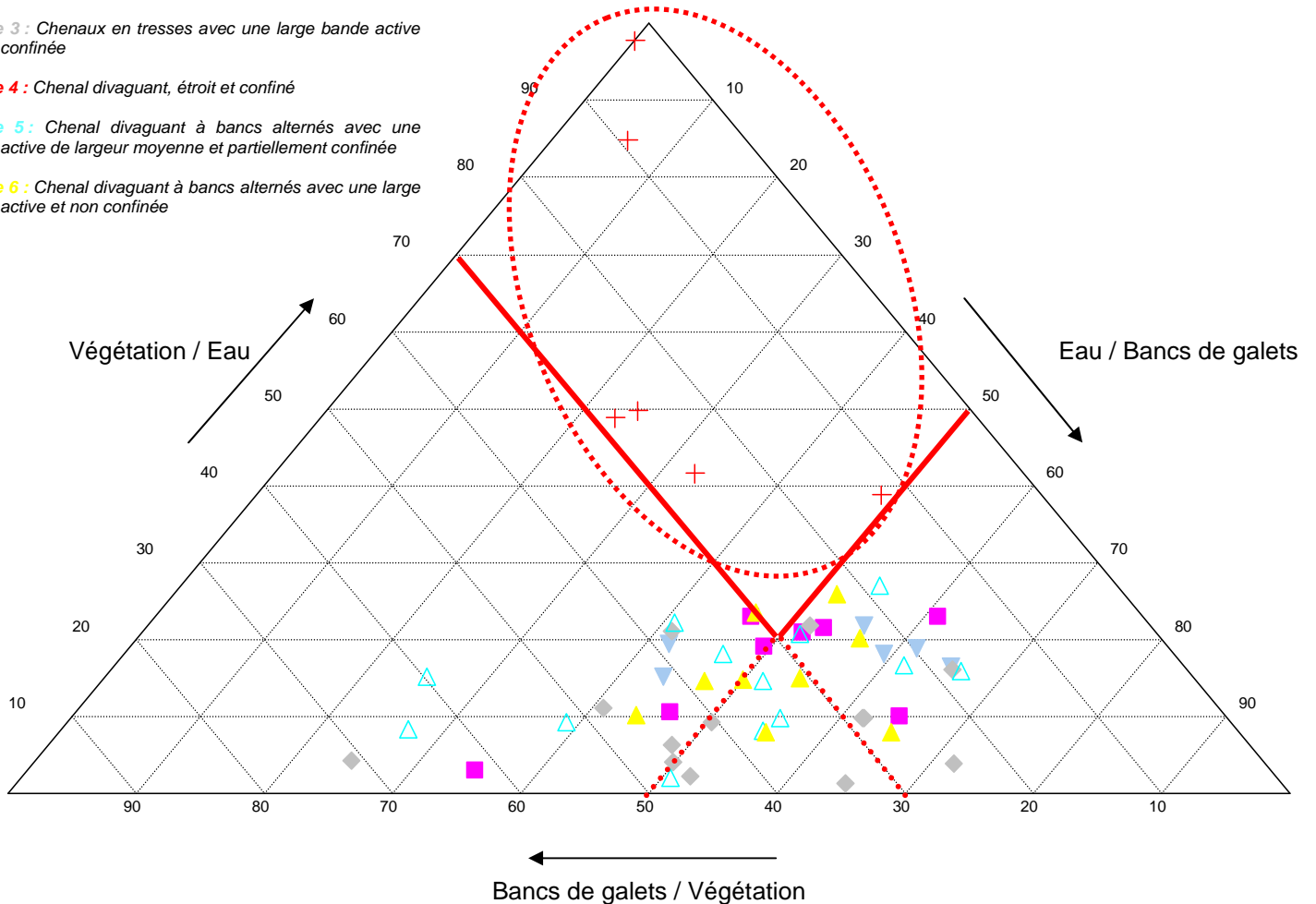
Figure 47: Graphique ternaire représentant les différents écotones présents dans le corridor alluvial en fonction du style fluvial
