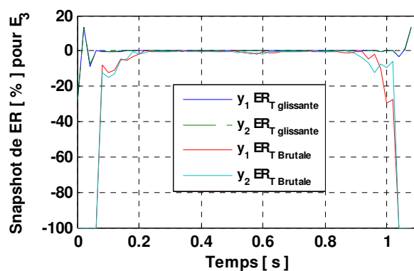
Figure 5. Les signaux de sortie et les erreurs relatives pour E_3
