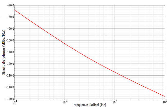
Figure 8. Bruit de phase simulé du réseau de VCO couplés pour \theta = 29^\circ .
