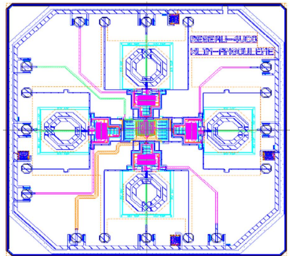
Figure 3. Dessin des masques du réseau constitué de quatre VCOs couplés.
