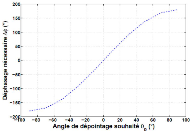
Figure 7. Déphasage en fonction de l'angle de pointage \theta_0 .
