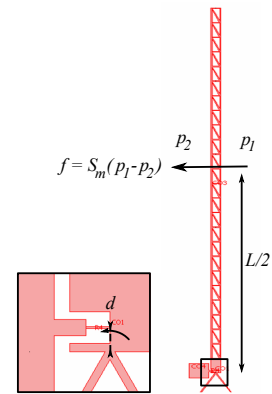
FIG. 4 – Effet de bras de levier assuré par les microstructures mécaniques.
