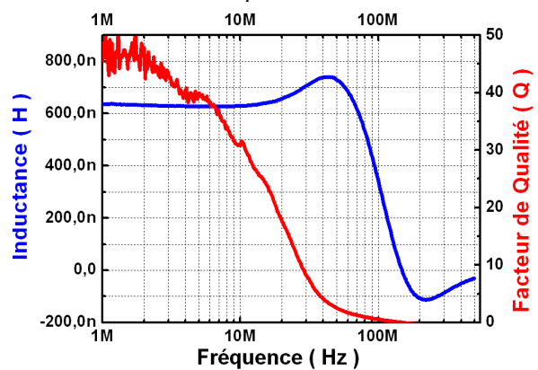
Fig 13. Mesures de l'inductance et du facteur de qualité d'un composant intégré en fonction de la fréquence.
