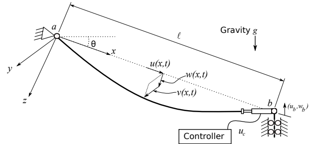
Fig. 1. Inclined Cable
