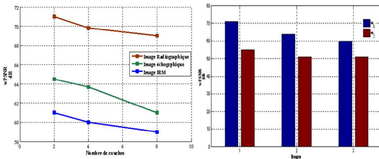
Figure 5. : (a) Mesure de la dégradation pour 2, 4 et 8 couches (b) Mesure de la dégradation de trois images tatouées avec deux coefficients de visibilité \alpha_1 (0.1) et \alpha_2 (0.5)
