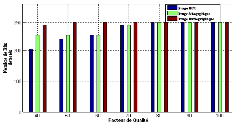
Figure 4. Nombre de bits détectés en fonction du facteur de qualité de la compression JPEG
