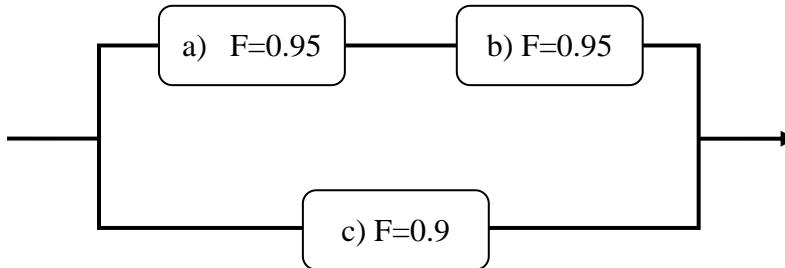
Schéma 2.2 Des éléments en série réduisent la fiabilité et accroissent le risque.
