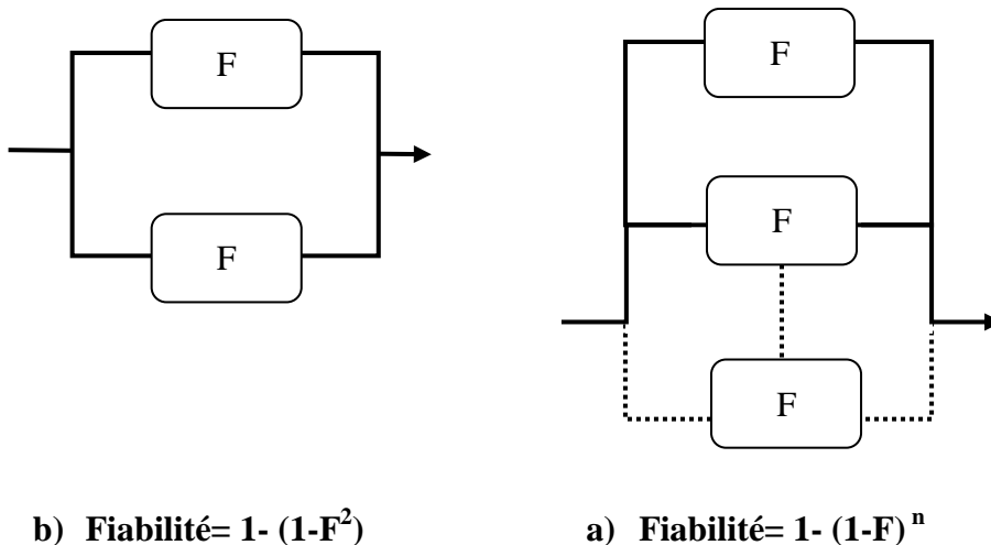
Schéma 2.1 Des éléments parallèles augmentent la fiabilité et diminuent le risque.
