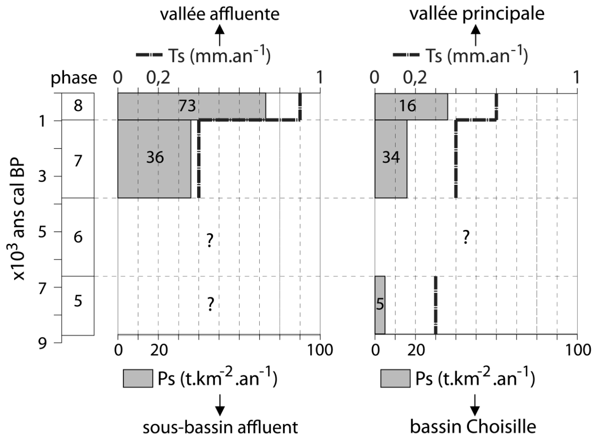
Figure 8 : Taux de sédimentation ( Ts en mm.an^{-1} ) et production sédimentaire solide minimale ( Ps en t.km^2.an^{-1} ) estimés d'après les stocks sédimentaires en fond de vallée – Sedimentation rates ( Ts in mm.an^{-1} ) and minimum solid sediment production ( Ps in t.km^2.an^{-1} ) estimated from sediment storage in the valley bottom.
