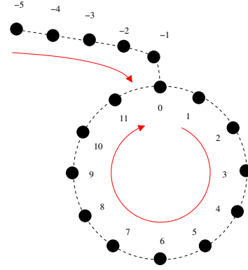
FIGURE 1: Une horloge bornée \mathcal{X} = (\text{cerise}(\alpha, K), \phi) avec \alpha = 5 et K = 12
