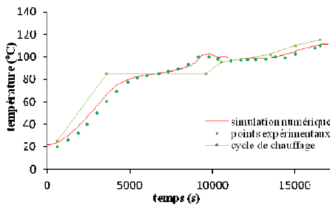
Fig. 10. Evolution de la température au centre d'un stratifié plan verre/polyester cuit en autoclave [7].
