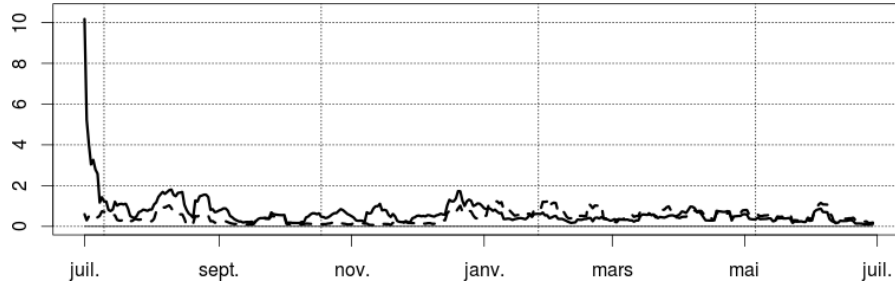
FIGURE 9. Dégradation moyenne du MAPE pour les deux configurations de perte de clients retenues, exprimée comme pourcentage du MAPE journalier sur la courbe sans pertes Efect .
