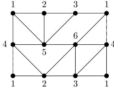
FIGURE 1 – Plongement de K_6 dans \mathbb{K}^2
