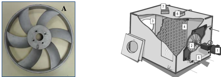
FIG. 1 – Vue du ventilateur A. Représentation du caisson aspirant ISO-5801. Dimensions : 1,3 \times 1,3 \times 1,8 m.
