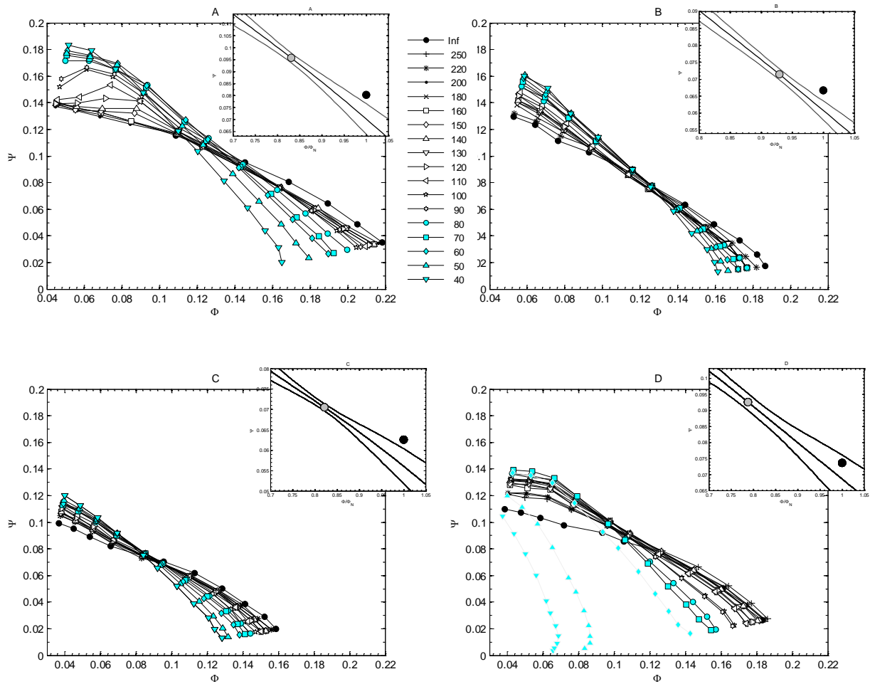
FIG.3 – : Influence de l'obstacle sur \Psi = f(\Phi) . Encarts : position relative du pivot et du débit nominal en champ libre ; la courbe moyenne ; les courbes \pm \sigma servant à la détermination systématique du pivot
