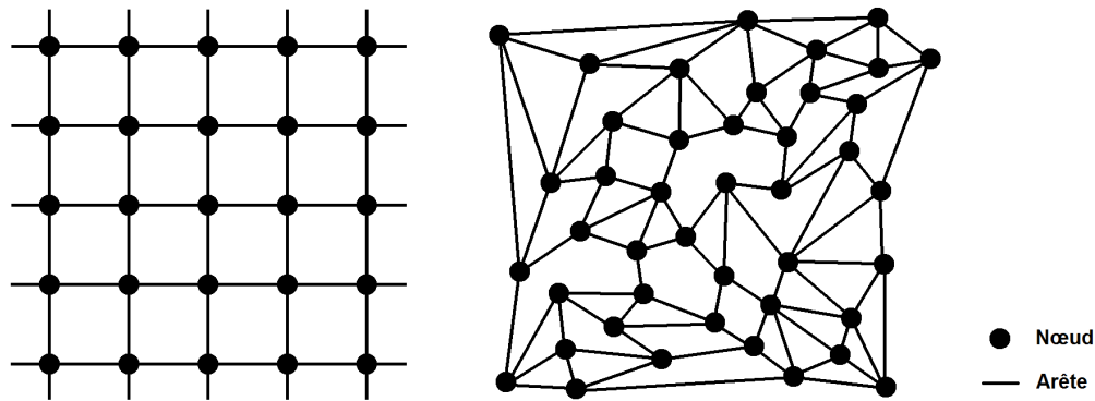
FIGURE 1: Tore (gauche) et graphe planaire 4-connexé (droite)
