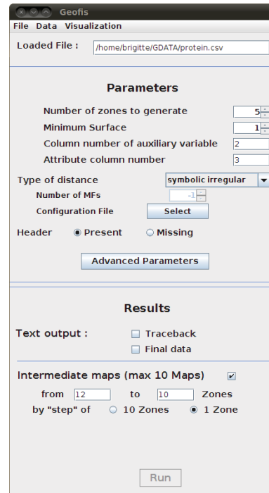
Fig. 7. GeoFIS zone learning parameters
