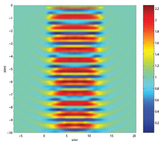
Figure 3: Coupe des isobars dans un plan vertical pour les x_3 < 0
