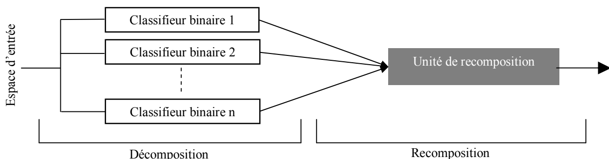
Figure 2 : classifieur décomposant le problème de classification en K classes en un ensemble de n classifieurs binaires ( N=K.(K-1)/2 ) dont les réponses sont traitées par l'unité de recombinaison qui sélectionne la réponse la plus pertinente.
