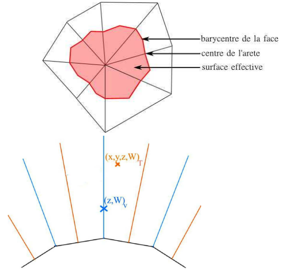
FIGURE 1 – Représentation schématique des normales au maillage au-dessus des sommets et des faces et de la surface effective associée à un sommet pour pondérer le nombre de multipliers associés à ce sommet.
