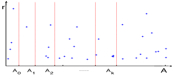
FIGURE 2 – Tirage des multiplieurs selon une loi approximativement uniforme à la surface du maillage et en 1/r^3 selon la normale : le nombre de multiplieurs attribués à un sommet k est proportionnel à la surface effective A_k de ce sommet.
