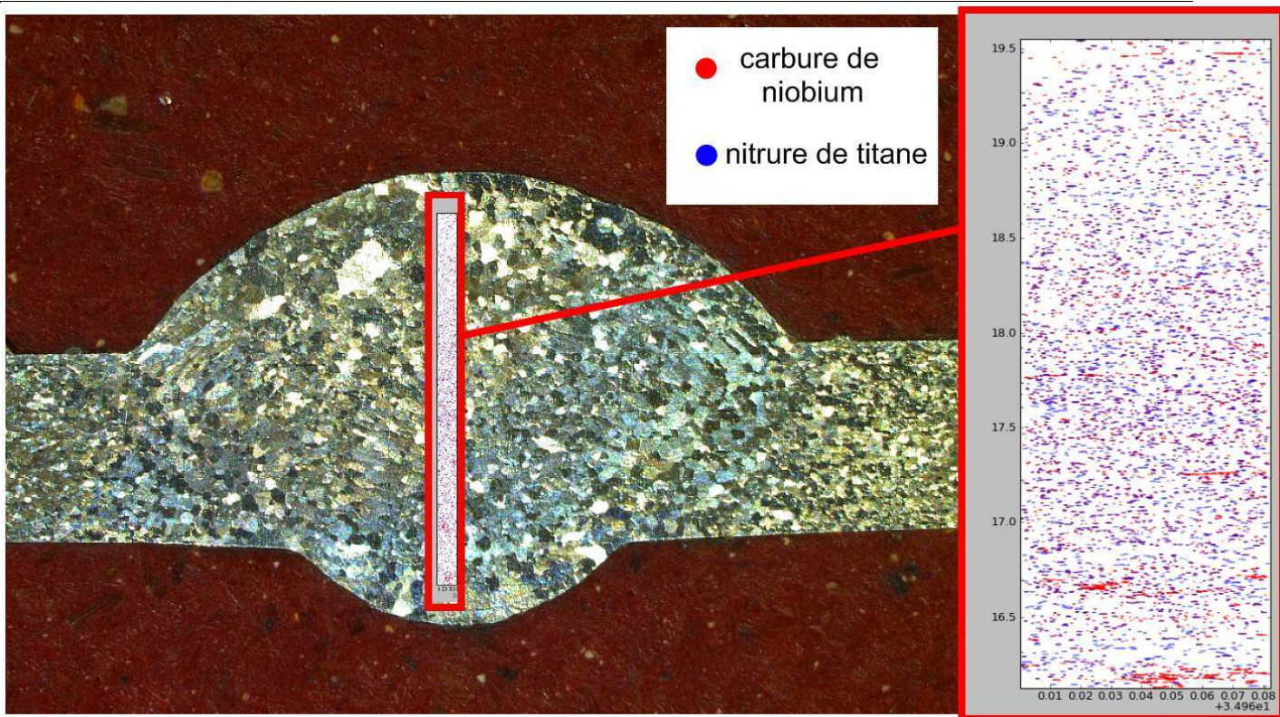
Figure 9 : exemple de répartition des précipités (K44-8 pulsé).
