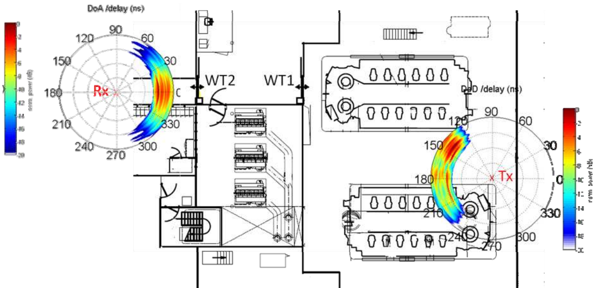
Figure 2 Résultats de mesure (diagramme coloré) d'un scénario de communication entre salles voisines dans les ponts inférieurs d'un ferry-boat.
