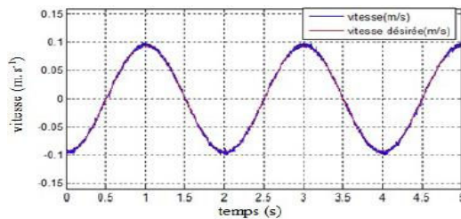
Fig.9. Vitesse désirée et estimée ( \text{m.s}^{-1} ) : DAO2
