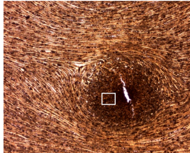
Figure 6: Vue d'une excroissance dans le plan transverse et du tissu ligneux l'entourant (dimension 4,10x3,03mm 2 )
