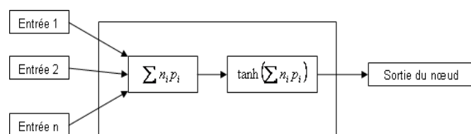
Figure 3 : Principe d'un nœud de réseau de neurones
