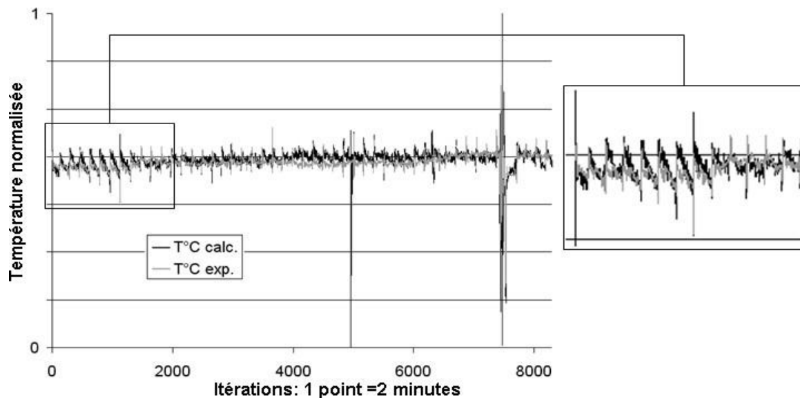
Figure 5 : Comparaison entre température expérimentale et température calculée
