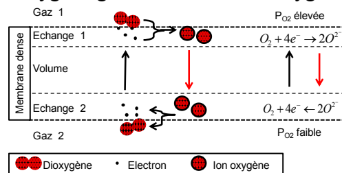
Figure 1 : Schéma des mécanismes de transport à travers une membrane
