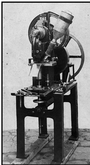
Machine à sabot circulaire
