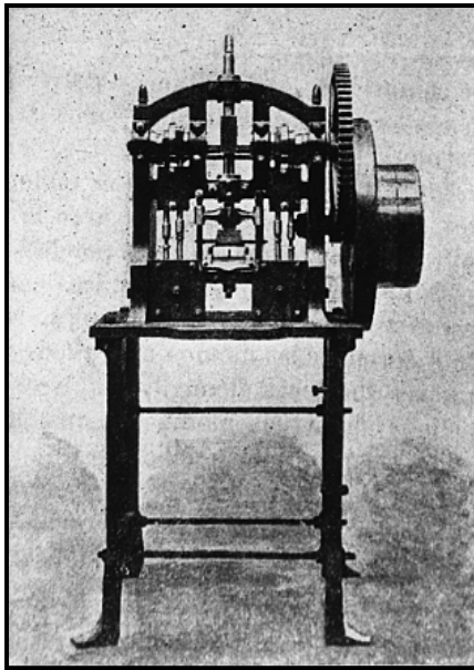
Machine alternative (d'après A .Andouard 1910)
