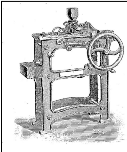
Presse Perfecta (d'après M.Bouvet)
