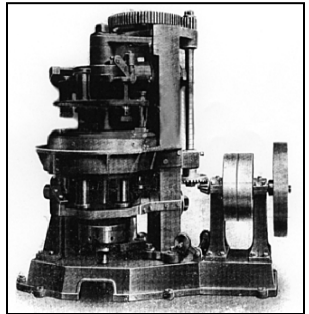
Machine rotative N°4
