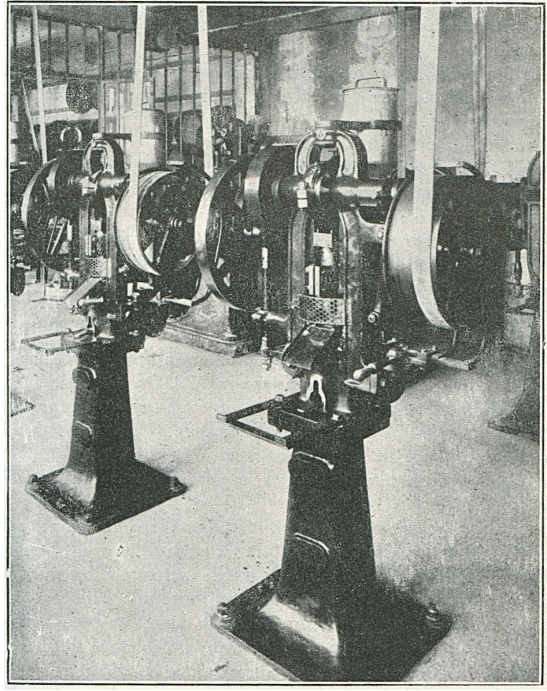
Atelier de compression des Etablissements David Rabot (Courbevoie- 1937) équipée de presses Frogerais N°0
