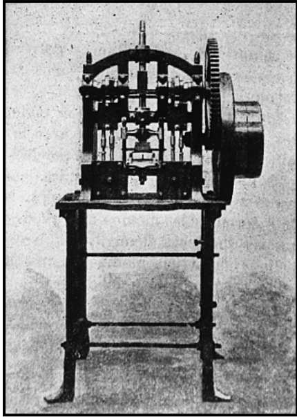
Machine alternative (d'après A. Andouard 1910)
