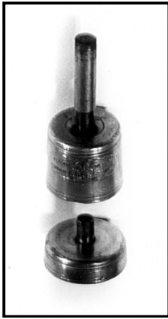
Appareils du type Brockedon fabriqué par May and Son (UK) - (4)
