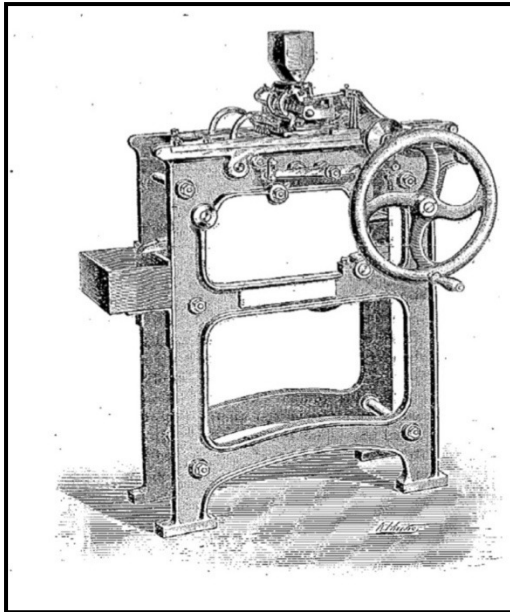
Presse Perfecta (d'après M. Bouvet)
