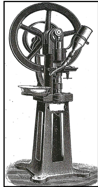
Machine L'IDEALE, version petit modèle et grand modèle (Catalogue Bachelet 1913)
