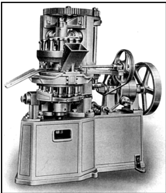
Machine rotative N° 3
