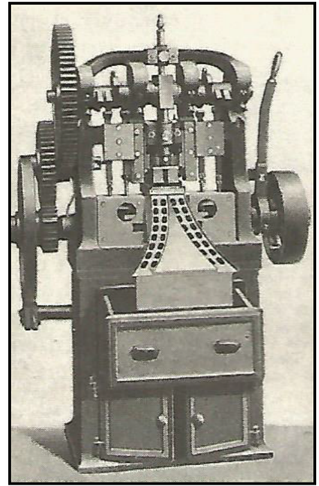
Machine Grand Modèle (1909)
