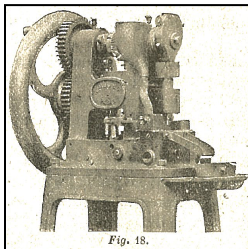
Machine alternative à sabot circulaire Palau (1892)
