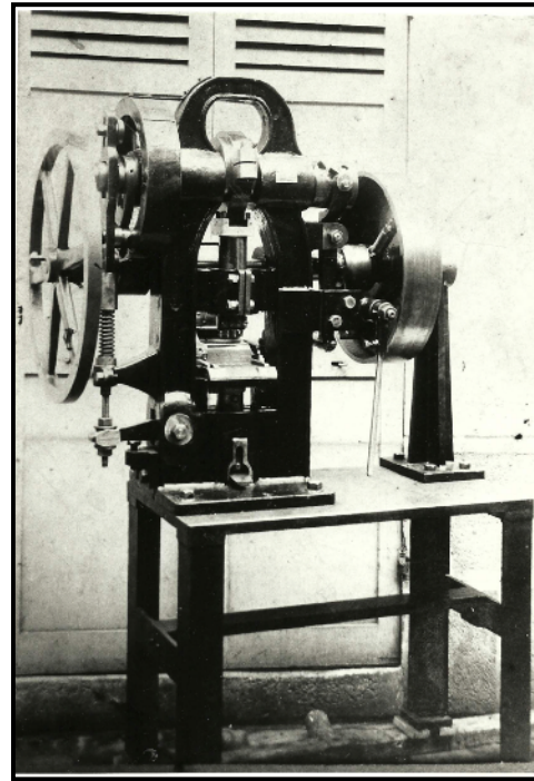
Machine à sabot linéaire
