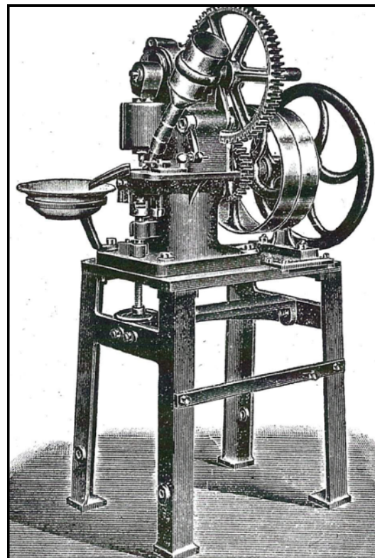
Machines petit et grand modèle Pouré (d'après M. Bouvet, 1919)
