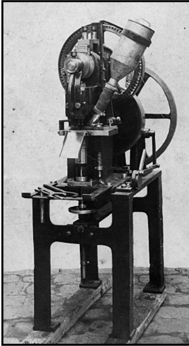
Machine à sabot circulaire
