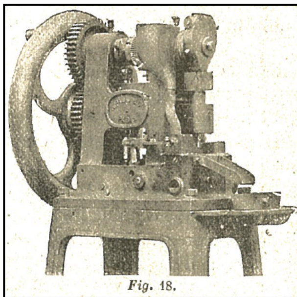
Machine alternative à sabot circulaire Palau (1892)
