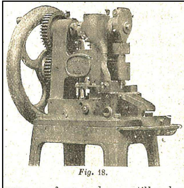
Machine alternative à sabot circulaire Palau (1892)
