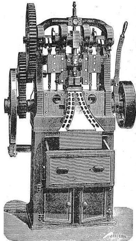
Machine alternative de production (d'après M.Bouvet 1919)
