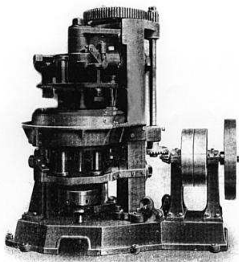
Machine rotative N°4
