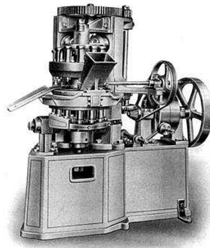
Machine rotative N°3
