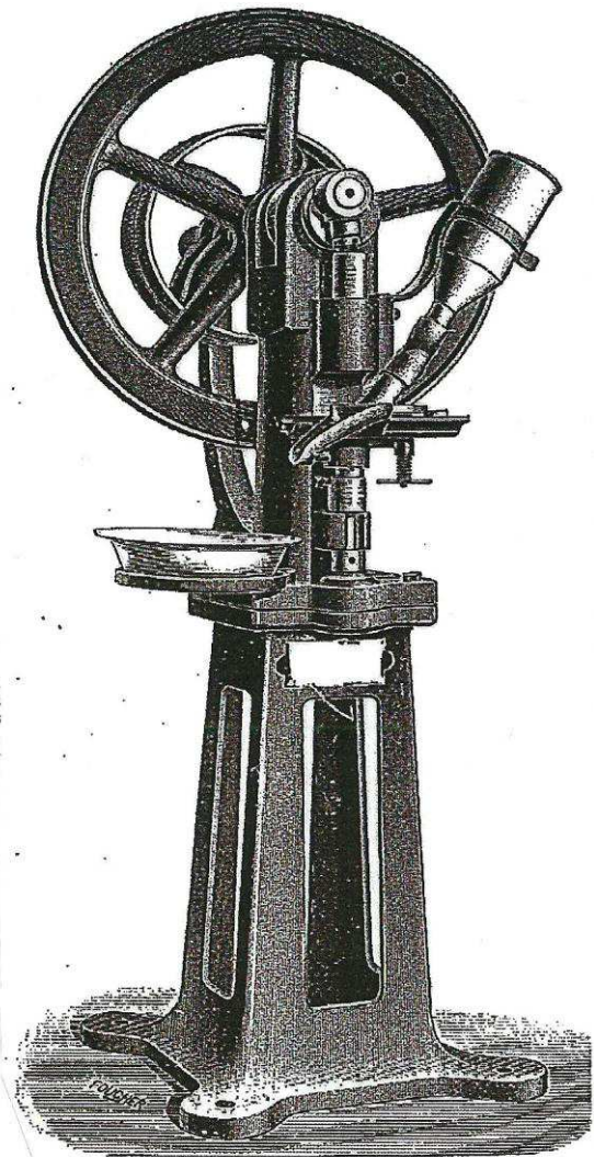
N° 8312 et 8313 Machine à comprimer « l'Idéale » grand modèle.
