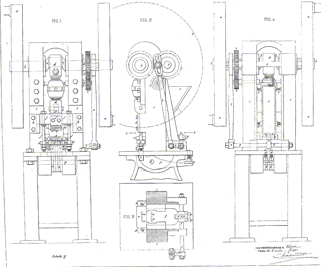
H. NÈGRE - MACHINE À COMPRIMER LES PRODUITS PHARMACEUTIQUES OU AUTRES SOUS FORME DE TABLETTES
