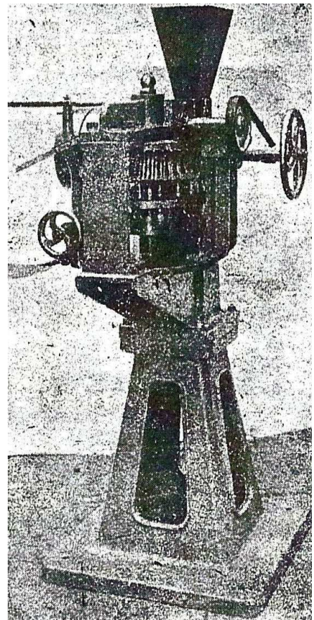
Machine à comprimer rotative Ratti dite « revolver » (d'après M.Bouvet)
