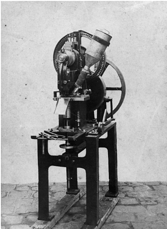
Machine à sabot circulaire
