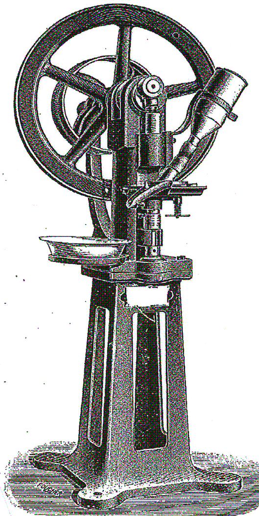
N° 8312 et 8313 Machine à comprimer « l'Idéal » grand modèle.
