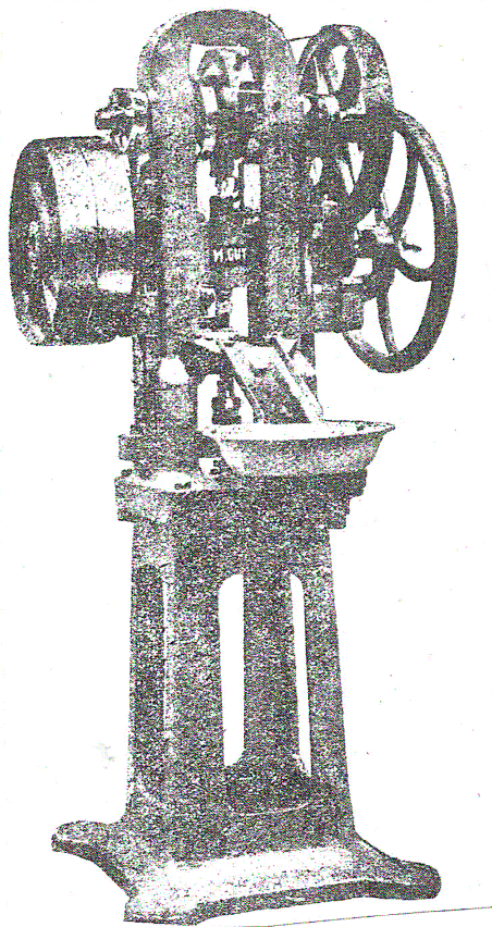
N° 8314-8315. — Machine à comprimer « l'Idéal », petit modèle. Cette machine est la même que le N° 8312, comme construction et comme production, mais la grosseur de la pastille ne doit pas dépasser 13 \frac{1}{2} .
