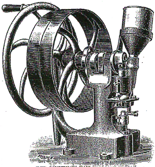
N° 8314-8315. — Machine à comprimer « l'Idéale », petit modèle. Cette machine est la même que le N° 8312, comme construction et comme production, mais la grosseur de la pastille ne doit pas dépasser 13 \frac{1}{2} .
