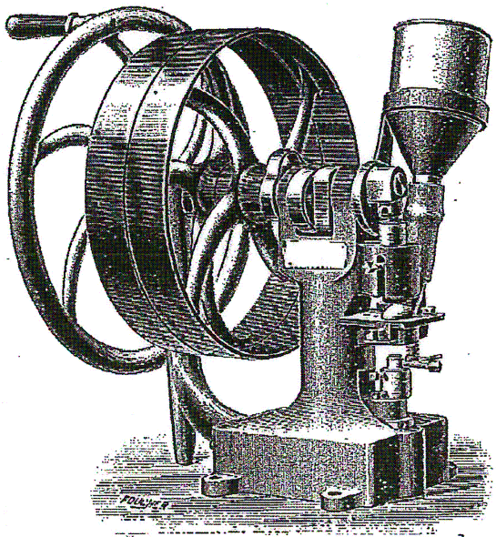
N° 8314-8315. — Machine à comprimer « l'Idéal », petit modèle. Cette machine est la même que le N° 8312, comme construction et comme production, mais la grosseur de la pastille ne doit pas dépasser 13 \frac{1}{2} .
