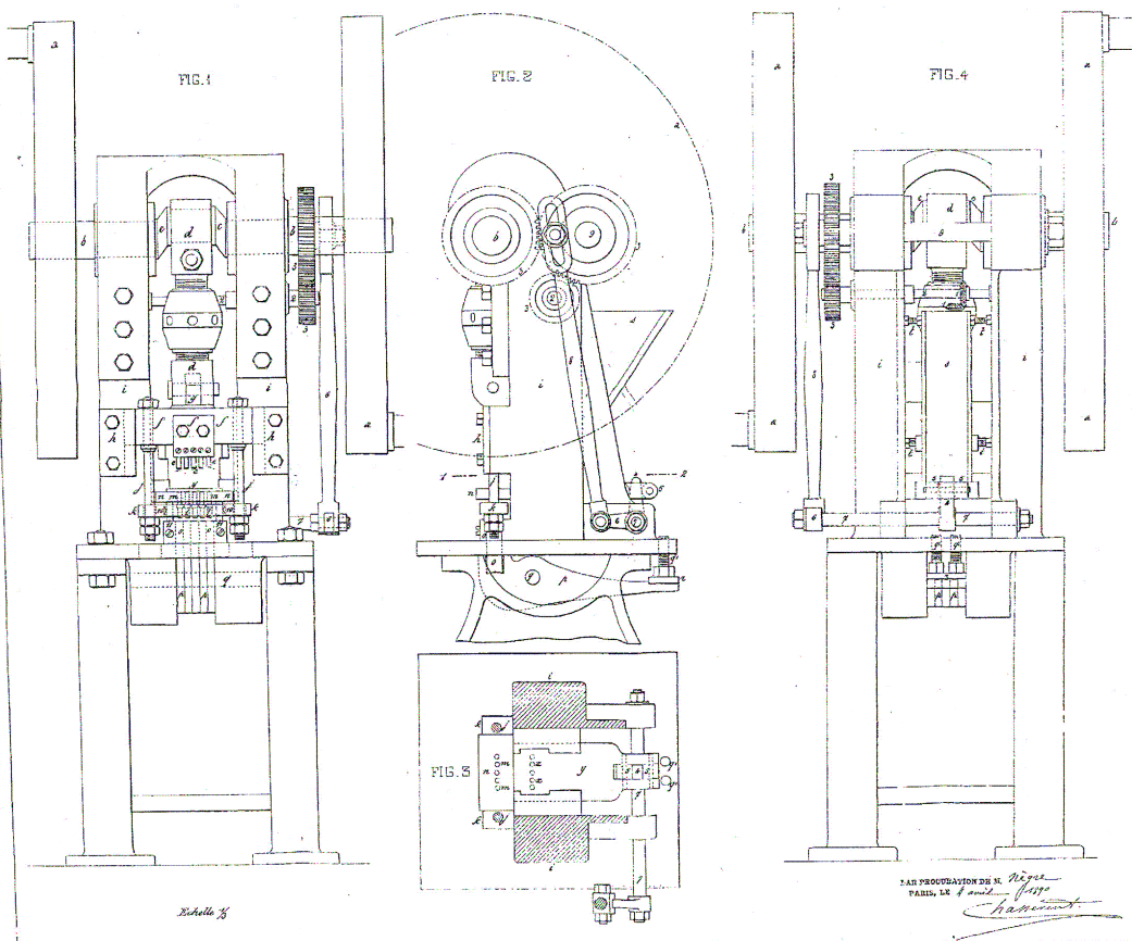
H. NEGRE - MACHINE A COMPRIMER LES PRODUITS PHARMACEUTIQUES OU AUTRES SOUS FORME DE TABLETTES
