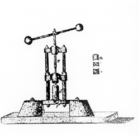
La presse de Rosenthal
