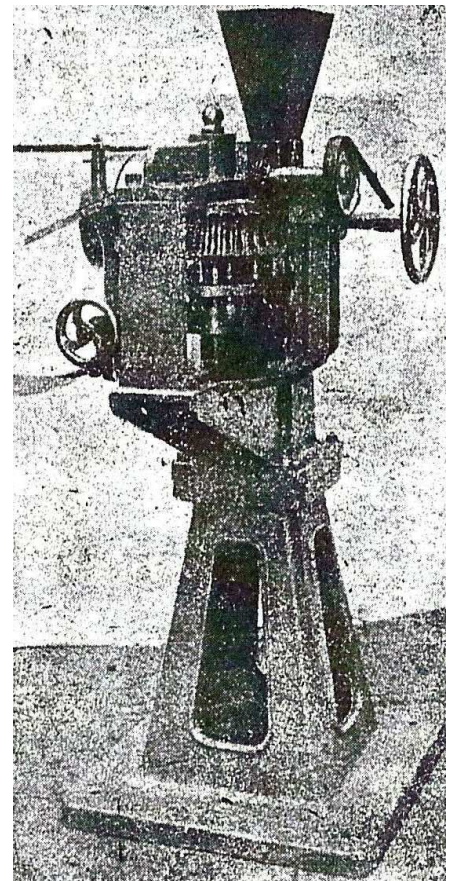
Machine à comprimer rotative Ratti dite « revolver » (d'après M.Bouvet)
