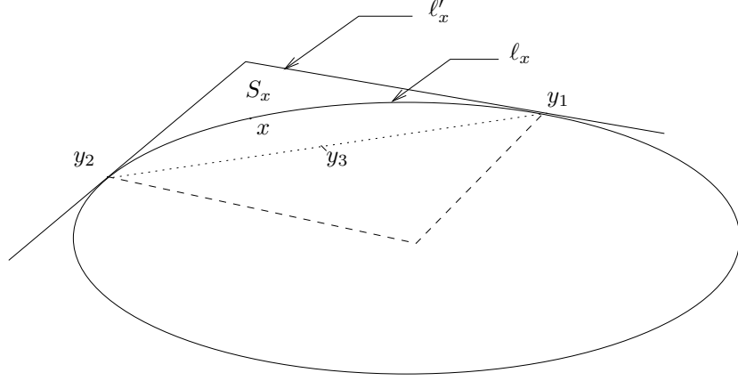
Fig. 2. The configuration in Lemma 1.
