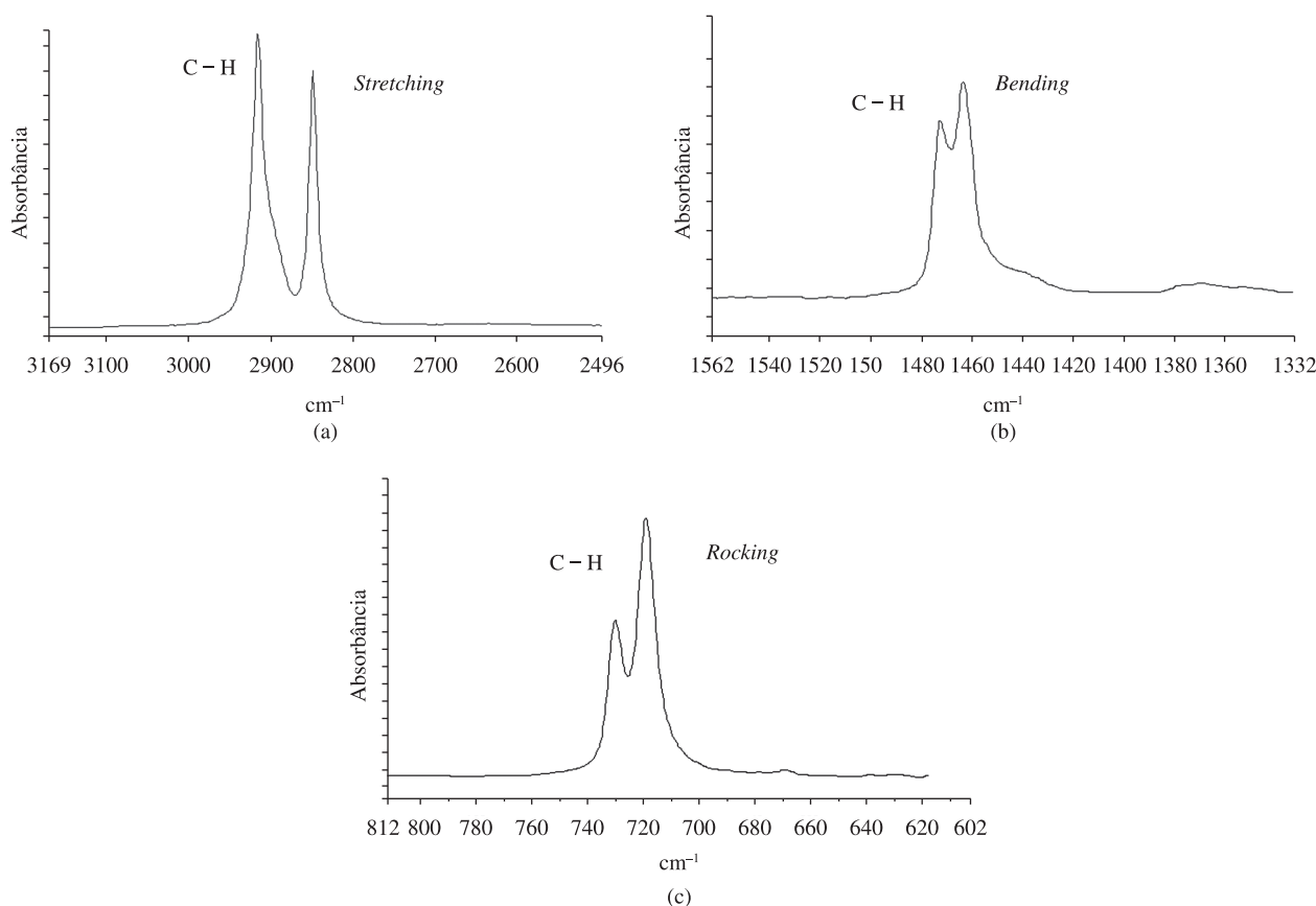
Figura 3. Detalhe das bandas de vibração das ligações C-H. a) Região entre 2500-3200 \text{cm}^{-1} ; b) região entre 1300-1550 \text{cm}^{-1} ; e c) região entre 600-800 \text{cm}^{-1} .
