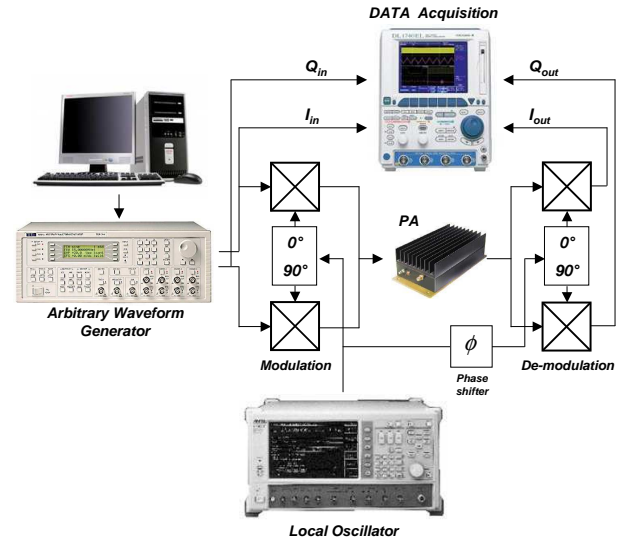
Fig. 3. PA setup
