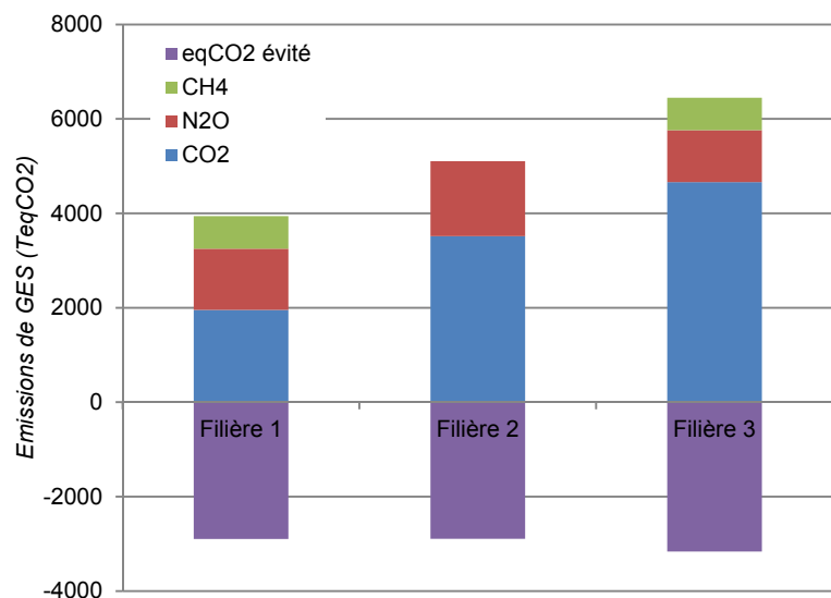
Figure III : Comparaison des émissions de GES en fonction de la nature du gaz pour les 3 filières
