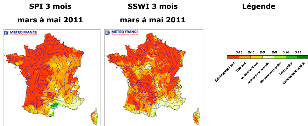
Figure 3 : cartographie de l'évolution de l'indicateur de sécheresse SPI et SSWI sur 3 mois en France en mai 2011 selon une représentation directement liée à la probabilité d'apparition du phénomène (durée de retour).
