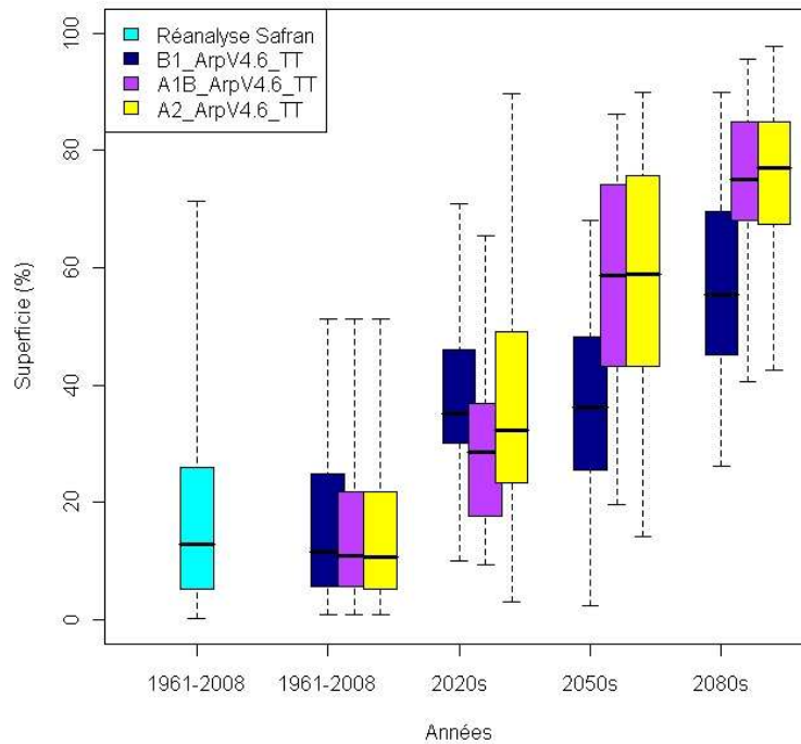
Figure 5 : même graphique que la figure 7 pour les sécheresses agricoles sur 3 mois (SSWI3).
