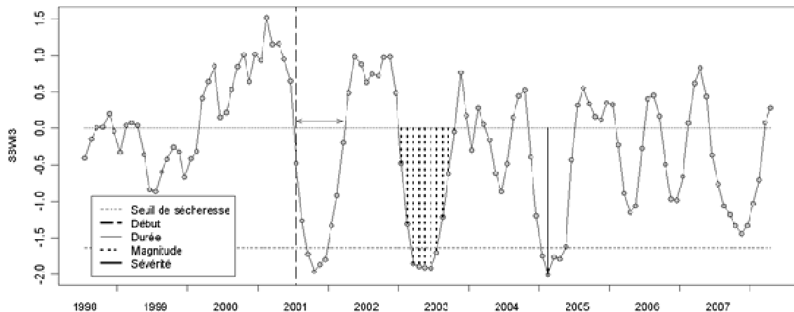
Figure 2 : définition des caractéristiques locales des événements de sécheresse : début, durée, magnitude et sévérité. Exemple de l'évolution du SSWI3 sur 10 ans sur une maille située près de Toulouse avec un seuil fixé à 5%.(source La Houille Blanche : DOI 10.1051/lhb/)
