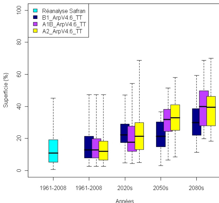
Figure 4 : diagramme en boîtes (valeur minimale, 1 er quartile, médiane, 3 e quartile et maximale) sur la période 1961 à 2100 pour la superficie affectée par les sécheresses météorologiques (SPI3), modérées à extrêmes, sur la France en fonction des scénarios climatiques B1, A1B, A2 du modèle ArpegeV4.6, régionalisation par type de temps (TT).
