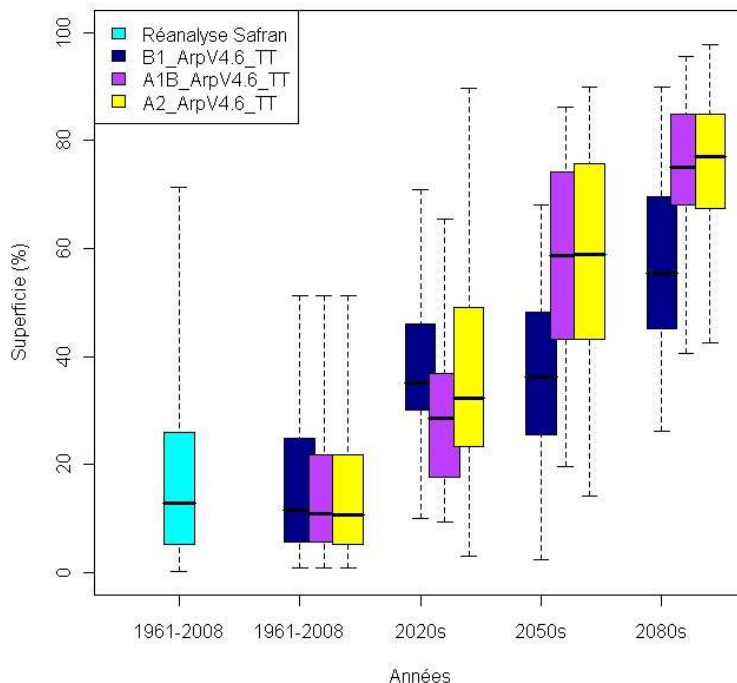
Figure 5 : même graphique que la figure 7 pour les sécheresses agricoles sur 3 mois (SSWI3).
