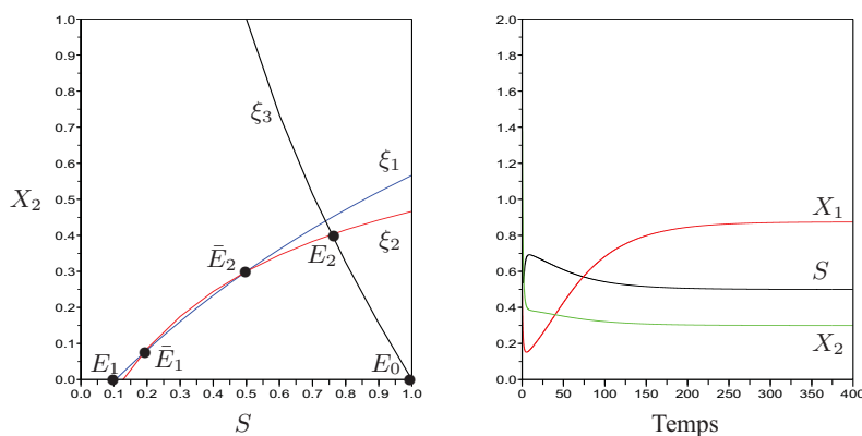
Figure 8. Bistabilité et coexistence
