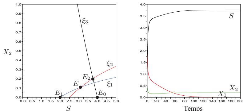
Figure 7. Exclusion compétitive de la première espèce par l'espèce la moins compétitive.
