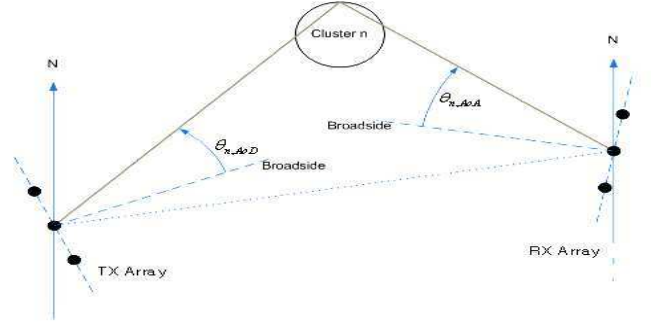
Figure 1 : Angular parameters : AOD/AOA
