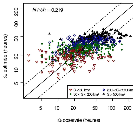
Figure 10 : Durées \theta_R observées et estimées selon la formule nationale
