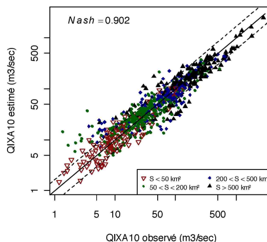
Figure 8 : Débits observés et estimés selon HER ( S, P_{24hXA10} )
