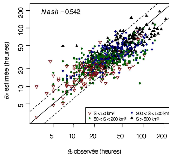
Figure 11 : Durées \theta_R observées et estimées selon HER (4 Var)
