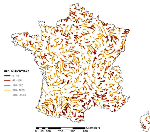
Figure 12 : Carte de \theta_R / (7,45 S^{0,27}) selon HER (4 Var) & Krigeage
