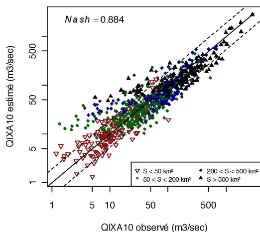
Figure 6 : Débits observés et estimés selon la formule nationale
