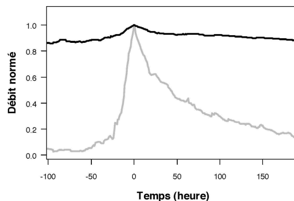
Figure 2 : Hydrogrammes de crue normés médians obtenus sur les débits (en noir) et sur les débits privés de la composante de base (en gris) de la Barbuise à Pouan-les-Vallées
