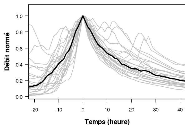
Figure 1 : Hydrogrammes normés (en gris) et hydrogramme médian (en noir) extraits de la série de débits privés de la composante de base de la Savoureuse à Giromagny
