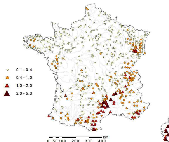
Figure 3 : Valeurs de QIXA10 spécifique aux stations de référence (en m 3 /s/km 2 )
