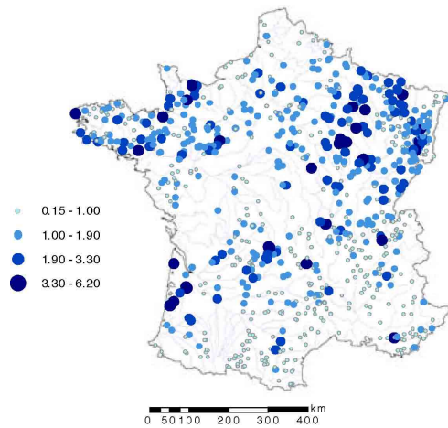
Figure 4 : Valeurs de \theta_R / (7,45S^{0,27}) aux stations de référence ( \theta_R en h, S en \text{km}^2 )
