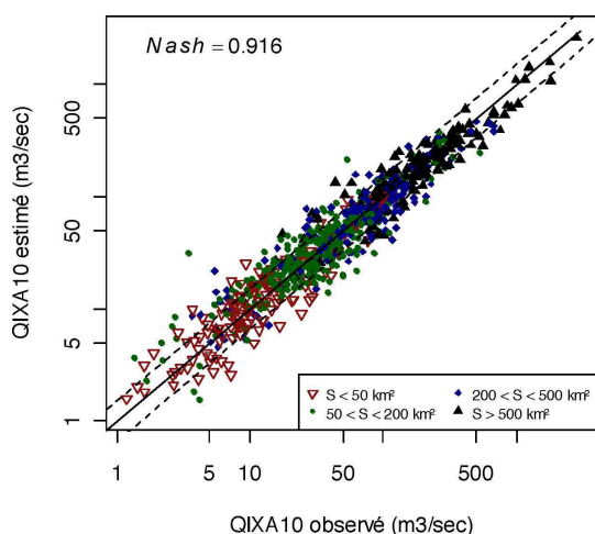
Figure 9 : Débits observés et estimés selon HER (4 Var)
