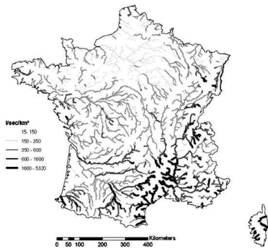
Figure 13 : Carte du QIXA10 selon HER (4 Var) & Krigeage
