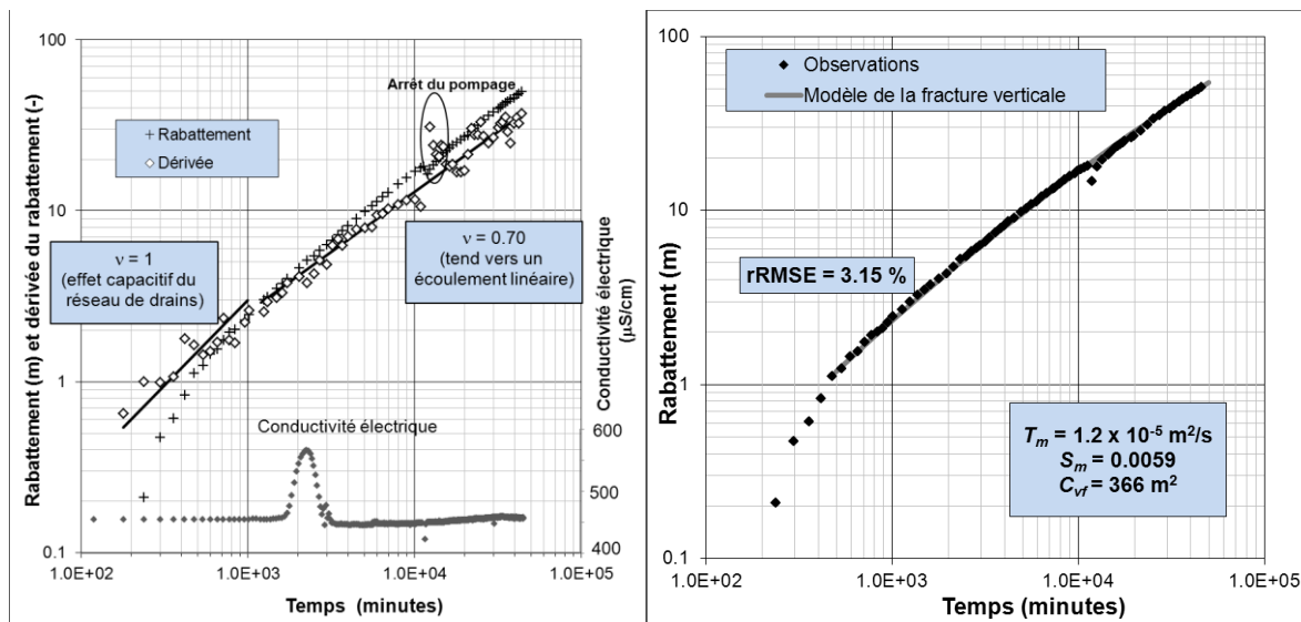
Figure 3: (a) Courbe diagnostique du pompage Cent-Fonts; (b) Evolution temporelle du rabattement mesuré et de sa modélisation par la solution de la fracture verticale (Ramey & Gringarten, 1976), modifié d'après Maréchal et al. , 2008
