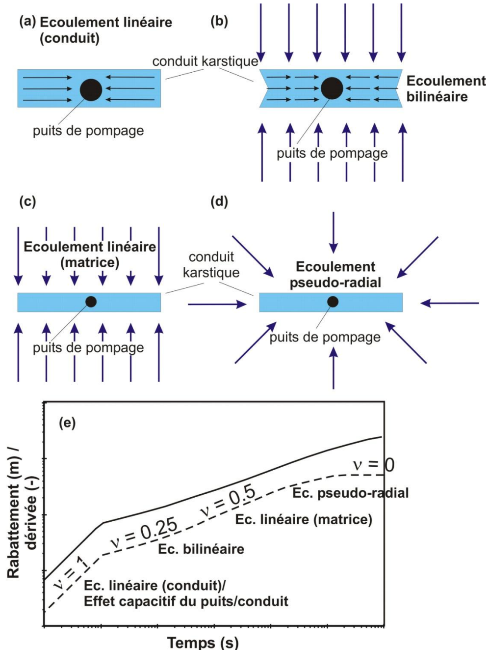
Figure 2 : réponse d'un puits interceptant un conduit karstique se comportant comme une fracture vertical de longueur finie et de perméabilité finie: (a) Écoulement linéaire dans le conduit ou effet capacitif du puits/conduit aux temps courts; (b) Écoulements bilinéaires; (c) Écoulement linéaire dans la matrice; (d) Écoulement pseudo-radial dans la matrice au cours des
