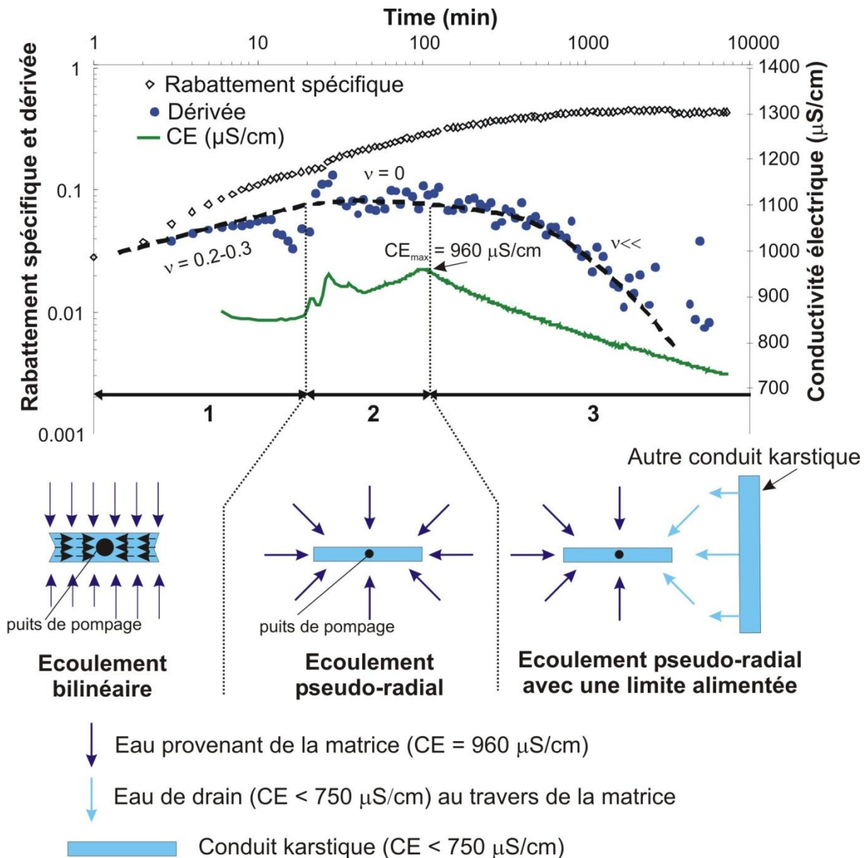
Figure 4 : essai de pompage au puits Robol, interceptant un petit conduit karstique profond
