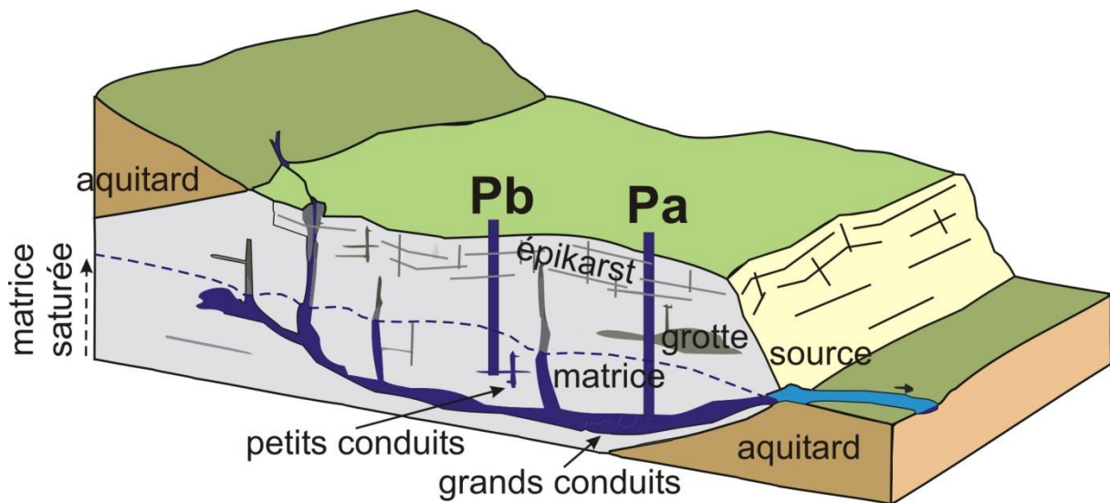
Figure 1 : aquifère karstique avec des puits de pompages (P) localisés au sein du réseau de conduits karstiques (modifié d'après Goldscheider & Drew 2007) – Pa : puits de pompage interceptant le réseau principal de drains karstiques, Pb : puits interceptant un petit conduit karstique
