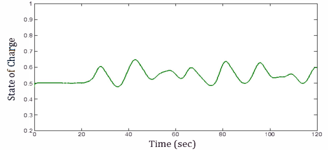
Fig. 17. Supercapacitor SoC.
