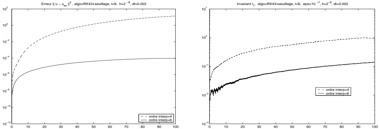
FIGURE 4. A gauche, évolution de l'erreur sur la solution \|u - u_{ex}\|_{L^2}^2 ; à droite, évolution de l'erreur relative E_1(t) pour des interpolations d'ordre 4 et 6.
