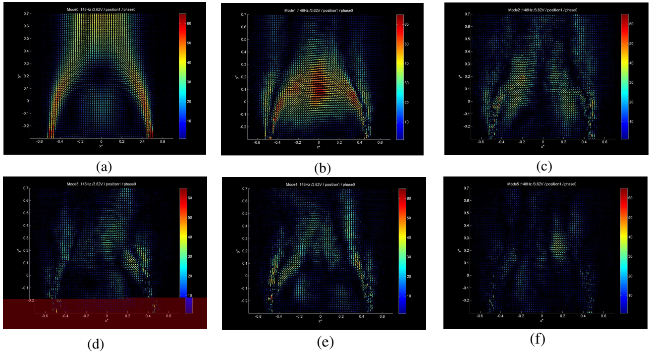
Fig. 5 P.O.D. analysis of a natural annular jet : (a) mode 0, (b) mode 1, (c) mode 2, (d) mode 3, (e) mode 4, (f) mode 5.
