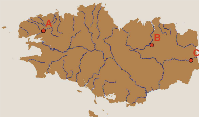
2 Résultats d'analyses ponctuelles d'isoproturon entre 2001 et 2006 dans l'Elorn à Pont-Ar-Bled (station A), à la retenue de Rophemel sur la Rance (station B) et au barrage de la Valière (station C).
