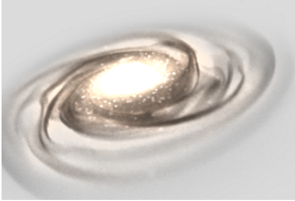
Figure 15: Projet ANR RTIGE : visualisation de galaxies
