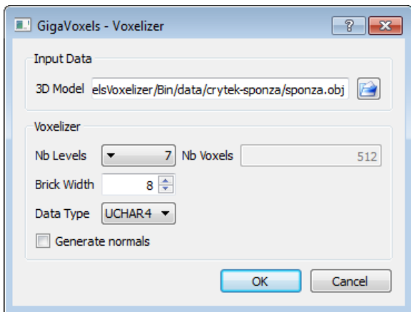
Figure 16: Voxeliseur GigaVoxels
