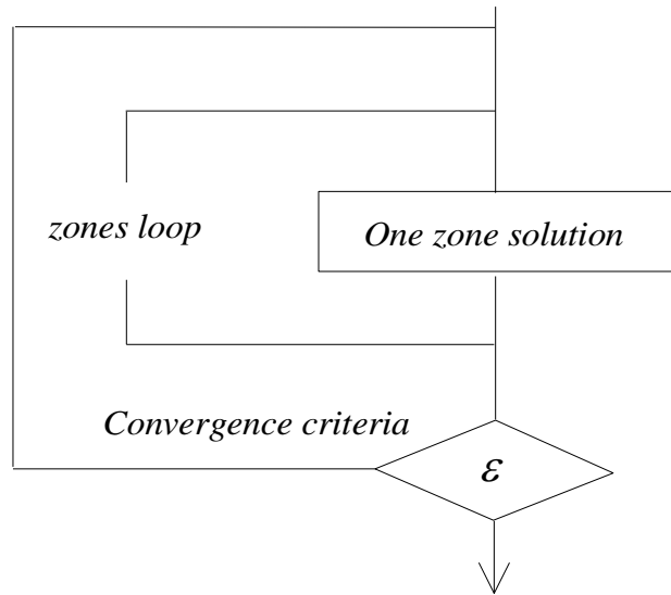
Fig. 7 : Coupling flowchart
