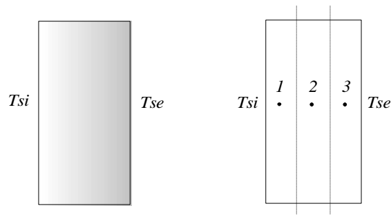
Fig. 2 : Wall spatial discretisation
