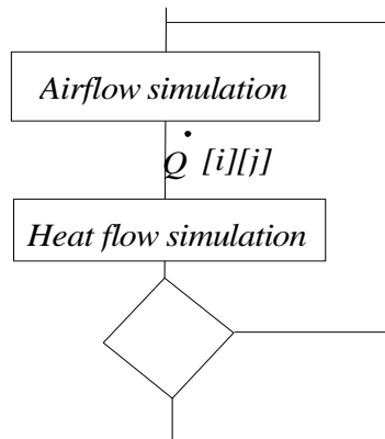
Fig. 3 : Coupling flow chart
