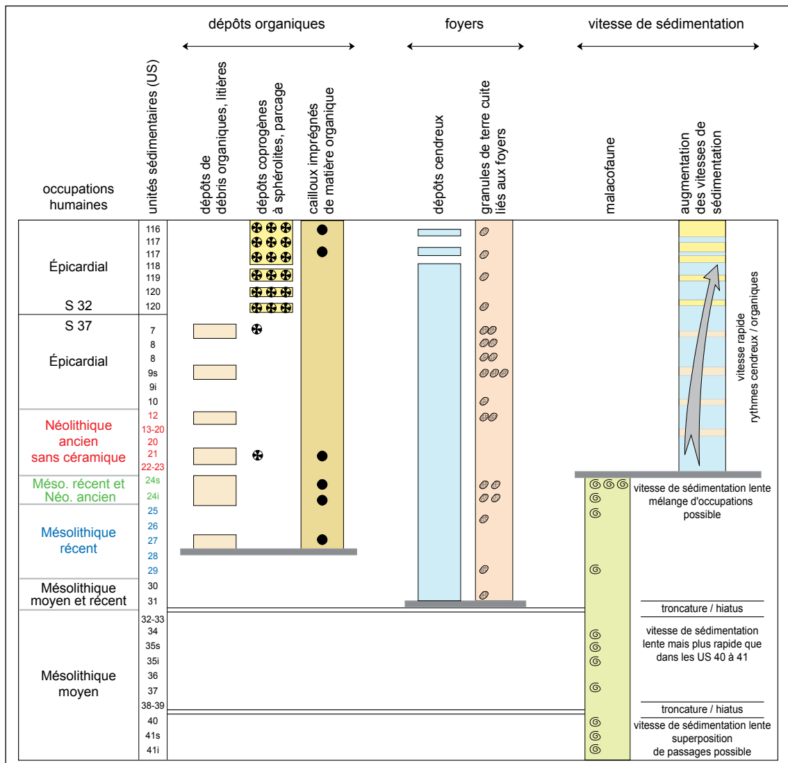
Figure 11 — Résultats principaux de l'analyse au microscope des sédiments du Mésolithique moyen au Néolithique ancien épicaldial (coupe stratigraphique S37 et S32 base). DAO : J. L. Brochier.
